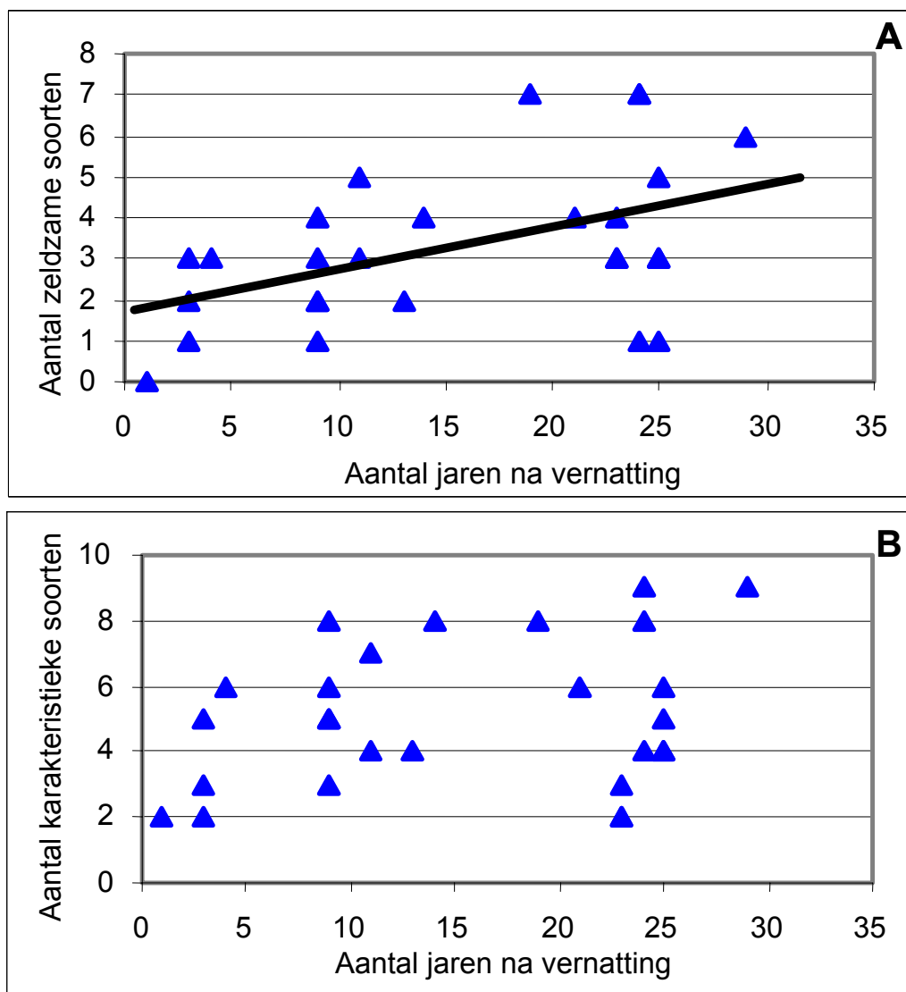
Figuur 26. Relatie tussen het aantal soorten en het aantal jaren na vernatting voor zeldzame soorten (a) en karakteristieke soorten (b) (naar: Van Duinen et al., 2003).
